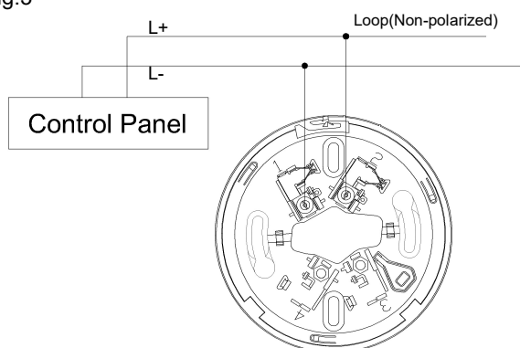
Fig.3. Loop wiring
